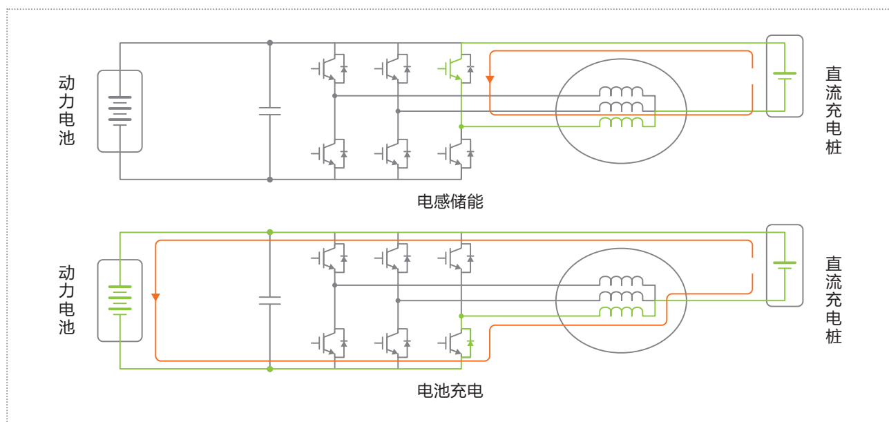
图 5 电驱动升压方案拓扑
