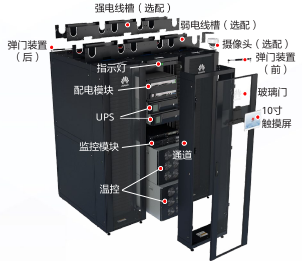
FusionModule800分解图
